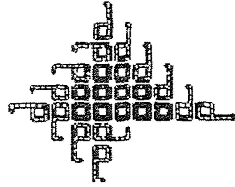
automate cellulaire autoreproductif
